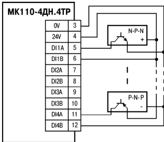
Рисунок Б.6 - Схема подключения к МК110-220.4ДН.4ТР дискретных датчиков с транзисторным выходом р-н-р-типа и н-р-н-типа с ОК (пример)
