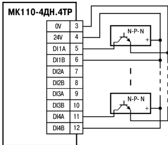
Рисунок Б.4 - Схема подключения к МК110-220.4ДН.4ТР дискретных датчиков с транзисторным выходом n-p-n-типа с ОК
