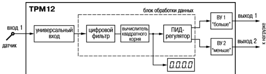
Рис. 3.1. Структурная схема прибора
