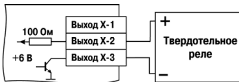
Рис. Б.4. Схема подключения к ВУ типа Т
