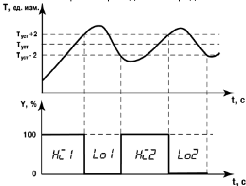
Рис. Е.1. АНР прибора, работающего в режиме нагревателя. Процесс АНР приведен на рисунке Е.1.
