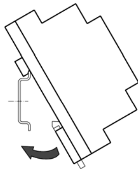
Рис. 5.3. Монтаж прибора с креплением на DIN-рейку
