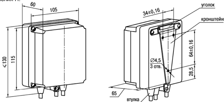
Рис. А.1. Прибор настенного крепления Н
