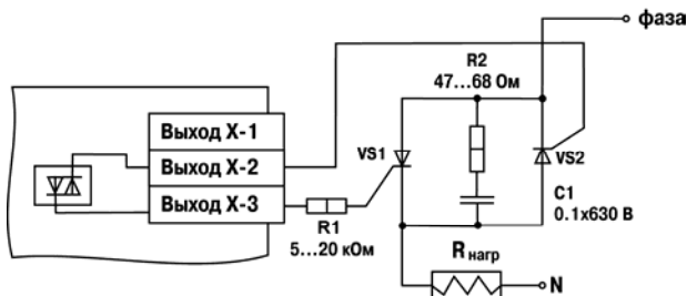
Рис. Б.4. Схема подключения к ВУ типа С двух тиристорov, подключенных встречно-параллельно
