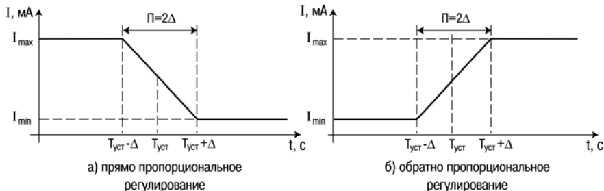
Рис. 3.13. Принцип формирования управляющего тока П-регулятора
