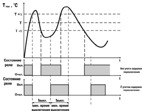
Рис. 3.12. Задание минимальных времен удержания выхода в замкнутом и разомкнутом состояниях для типа логики 1
