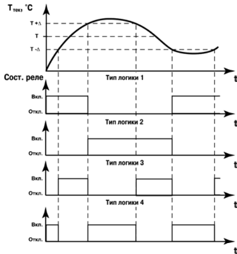
Рис. 3.10. Типы логики при работе ЛУ в режиме устройства сравнения
