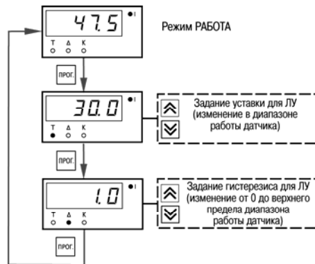
Рис. 6.1. Последовательность работы с прибором на первом уровне программирования
