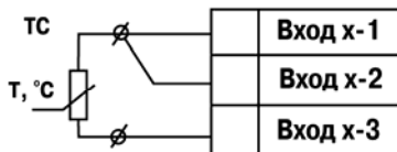
Рис. Б.9. Схема подключения термометра сопротивления
