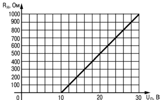
Рис 3.16. График зависимости R_H(U_n)
