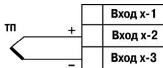
Рис. Б.10. Схема подключения термоэлектрического преобразователя
