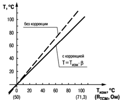
Рис. 3.4. Коррекция «наклон характеристики»
