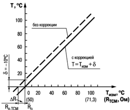
Рис. 3.3. Коррекция «сдвиг характеристики»
