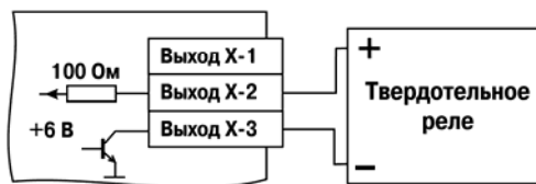
Рис. Б.8. Схема подключения к ВУ типа Т
