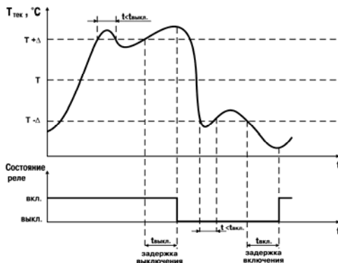
Рис. 3.11. Задание задержек включения/выключения ВУ для типа логики 1
