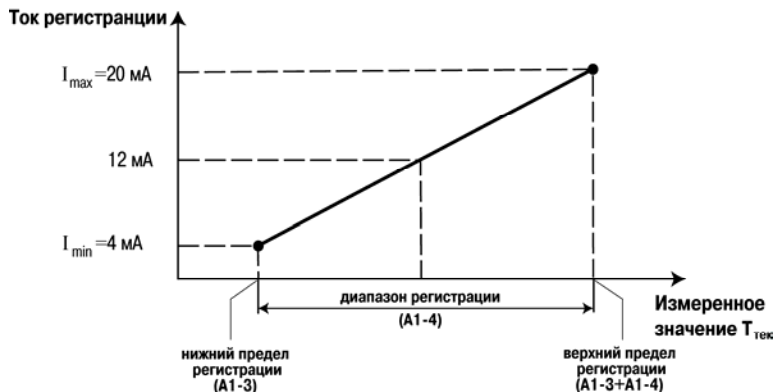
Рис. 3.14. Принцип формирования тока регистрации
